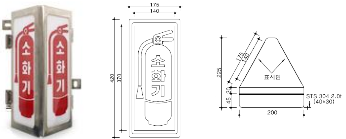
소화기 표시등
