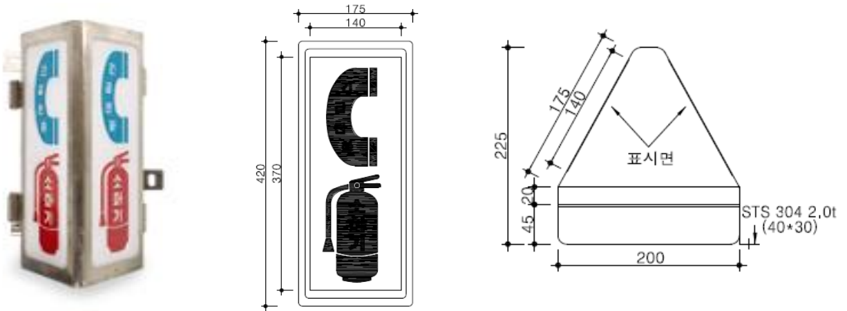
통합형 표시등
